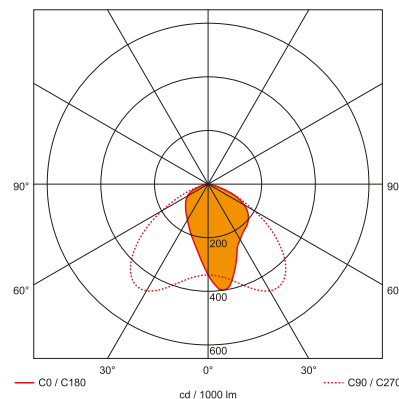
RHIS150 fényeloszlási görbe
