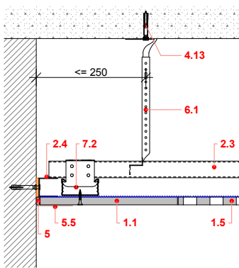
Hangelnyelő álmennyezetek dilatációja
