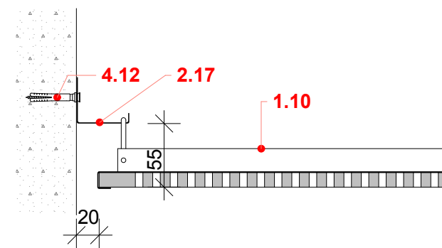
Gyptone Trap elem rögzítése a falhoz frízprofilal
