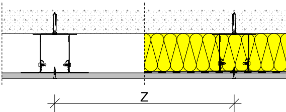
Általános részlet
