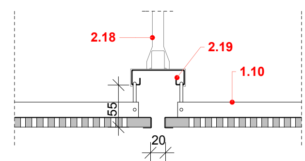
Gyptone Trap elemek csatlakozása közbenő profilhoz
