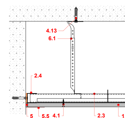
Hűtő-fűtő álmennyezet tartószerkezete Panelekkel párhuzamos metszet
