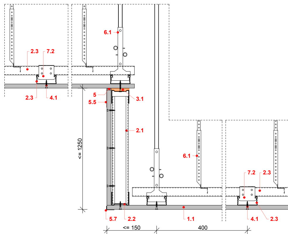
Álmennyezet lépcsőzése
