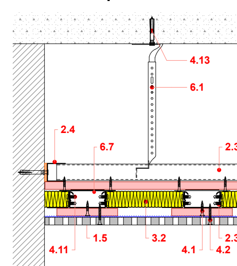
Tűzgátló és hangelnyelő álmennyezet falcsatlakozása – főtartókkal párhuzamos metszet
