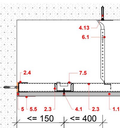
Falcsatlakozás UD-profillal
