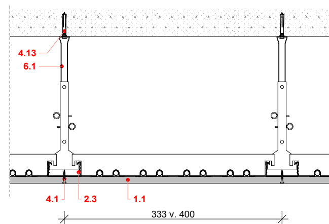
Hűtő-fűtő álmennyezet tartószerkezete Panelek merőleges metszet
