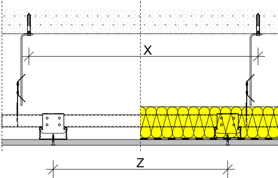
Általános részlet
