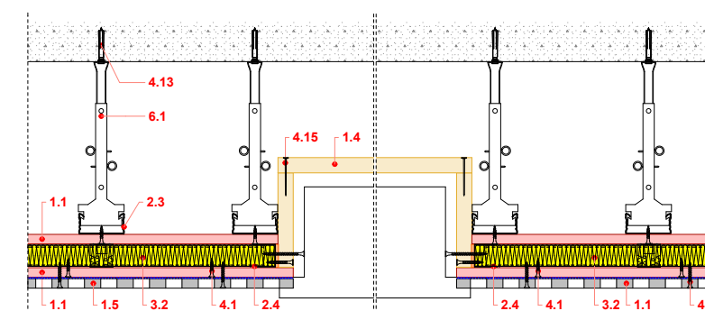
Lámpatest elhelyezése tűzgátló és hangelnyelő álmennyezetben, tűzvédelmi dobozolóval
