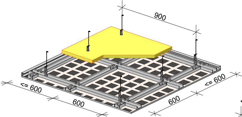
Gyptone nagytáblás
