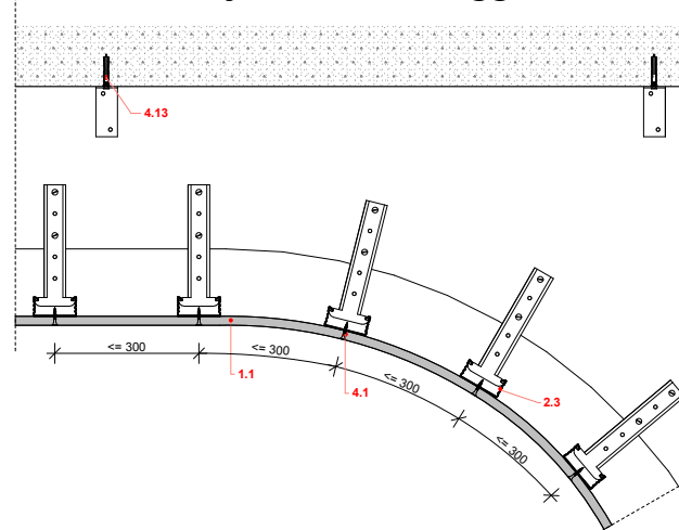
Íves álmennyezet merev függesztéssel
